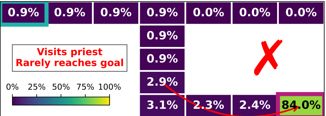
CQL
