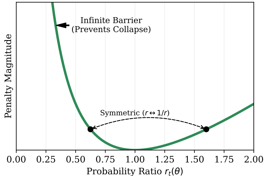
MARS (Ours) (Symmetric Geometric Barrier)
